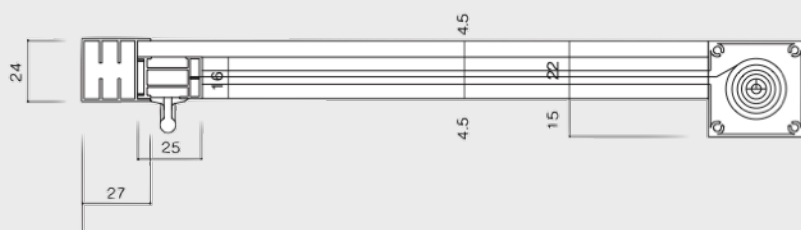
標準タイプ(ケース38×38)
