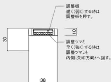
スリムタイプ(ケース38×38・18mmBタイプ)
